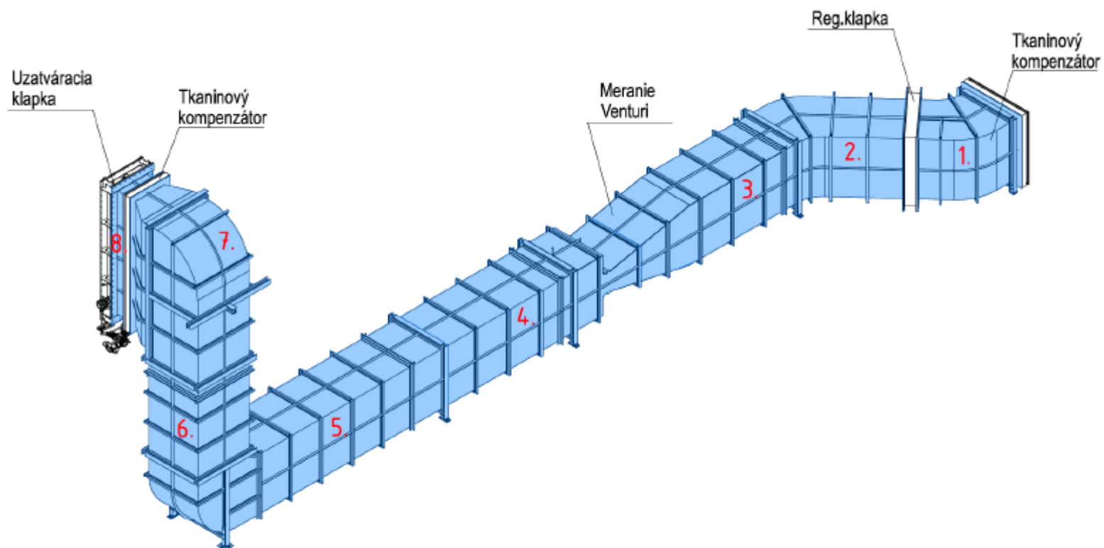
Obr. Potrubie recispalín
